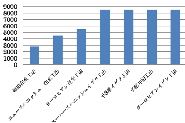
耐風圧試験結果（最大耐風圧力 (N/m 2 )
